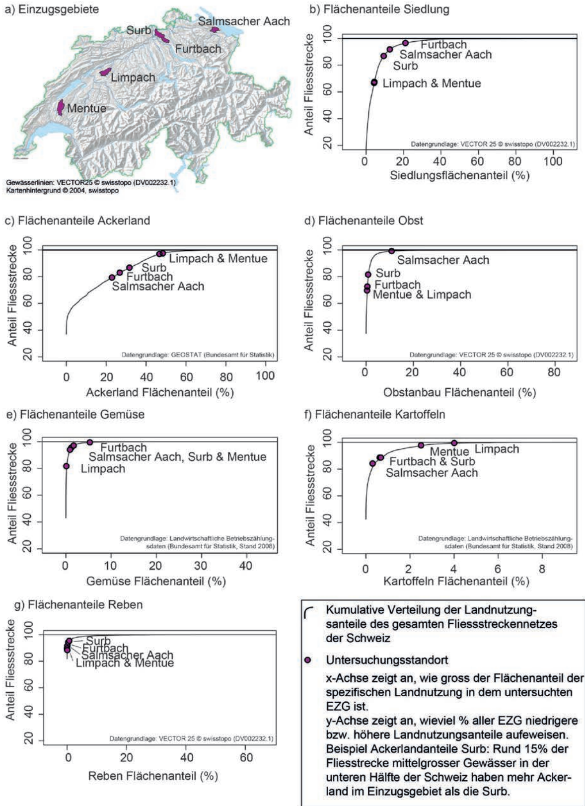
Fig. 1 a) Einzugsgebiete (EZG) der fünf ausgewählten Messstellen. b-g) Kumulative Landnutzungsanteile in den EZG der Flie遝sstrecken aller mittelgrossen Flie遝sgewässer (Flosz 3-6) b) kumulative Siedlungsflächenanteile, c) kumulative Ackerlandflächenanteile, d) kumulative Obstflächenanteile, e) kumulative Gemüseanteile, f) kumulative Kartoffelanteile, g) kumulative Rebenanteile a) Bassins versants (BV) des 5 points de mesure, b-g) Parts cumulatives d'utilisation du territoire (BV des voies d'écoulements de tous les cours d'eau de dimension moyenne) (Flosz 3-6), b) Somme des surfaces bâties, c) Sommes de surfaces cultivées, d) Somme des surfaces de verger, e) Sommes des surfaces maraichères, f) Somme des surfaces allouées à la culture de pommes de terre, g) Somme des vignes
